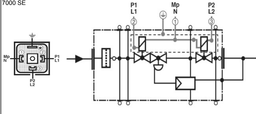
Электрическое подключение MBC-1900-7000 SE
